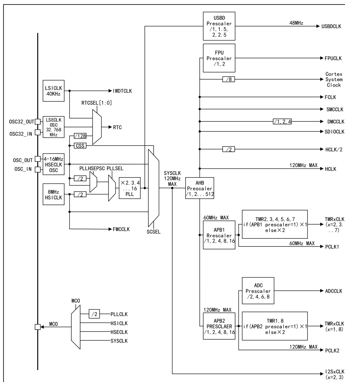
图 4 APM32A103xET7 时钟树
