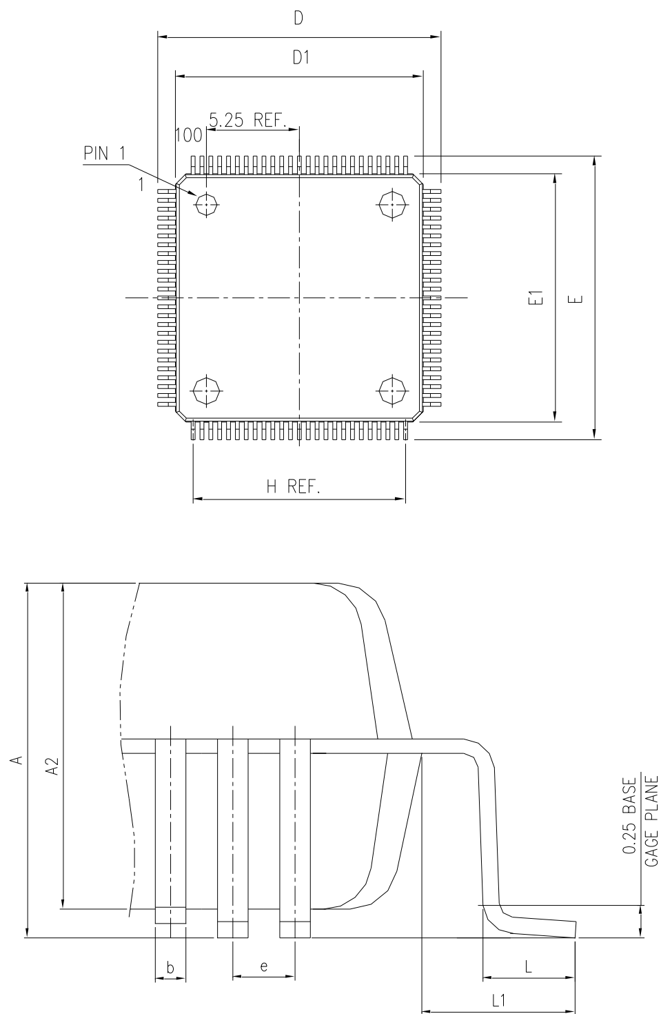
图 14 LQFP100 封装图
