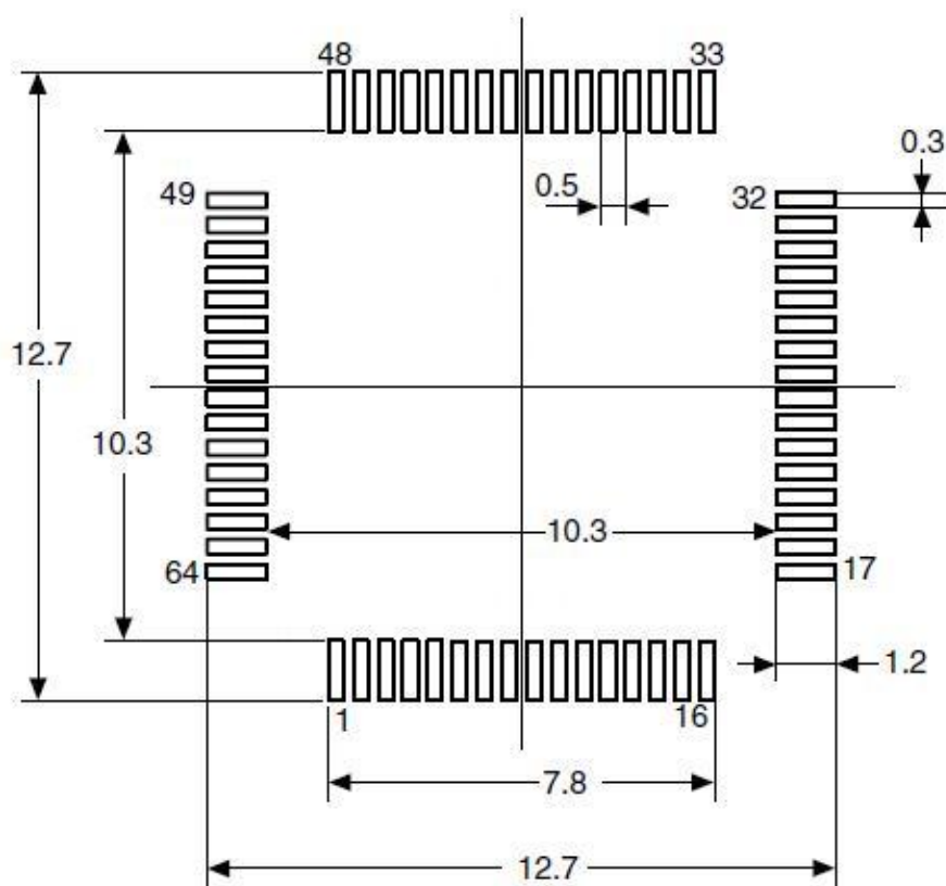
图 18 LQFP64 - 64 引脚，10 x 10mm 焊接 Layout 建议
