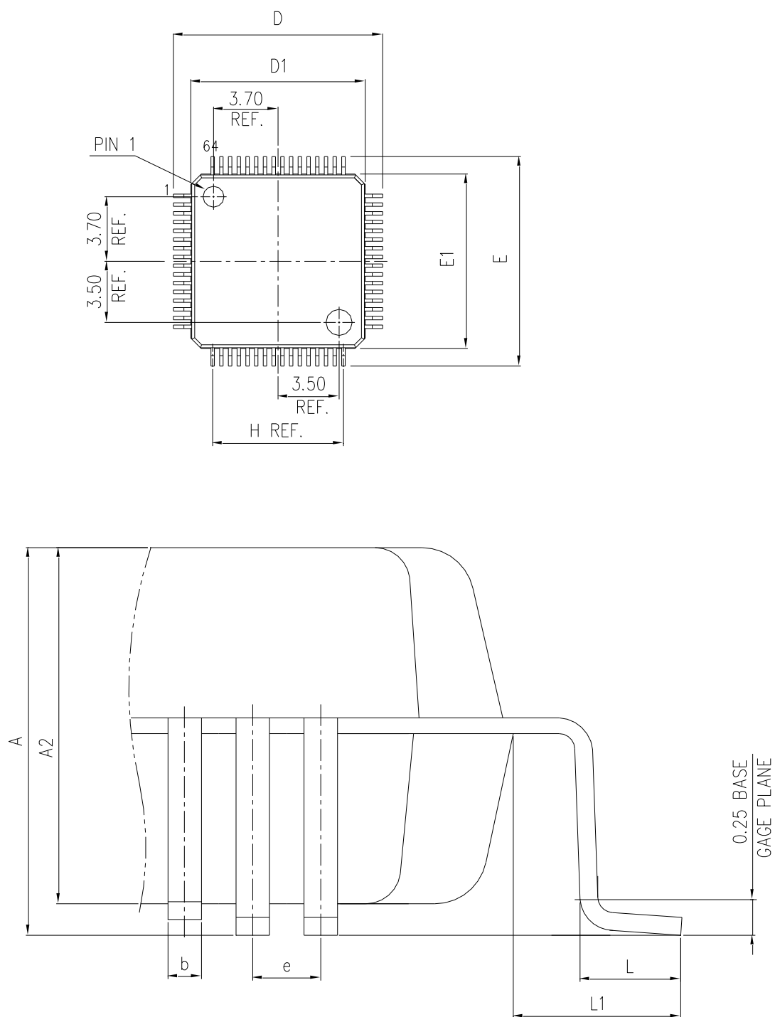
图 17 LQFP64 封装图
